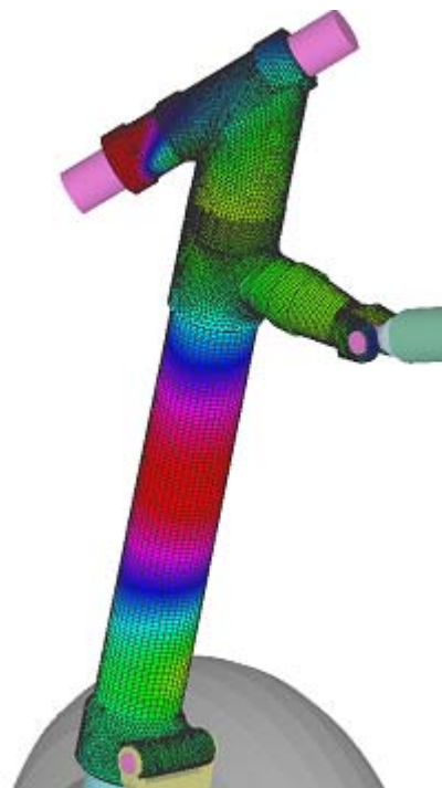
Рисунок 7. МКЭ-модель корпуса стойки
