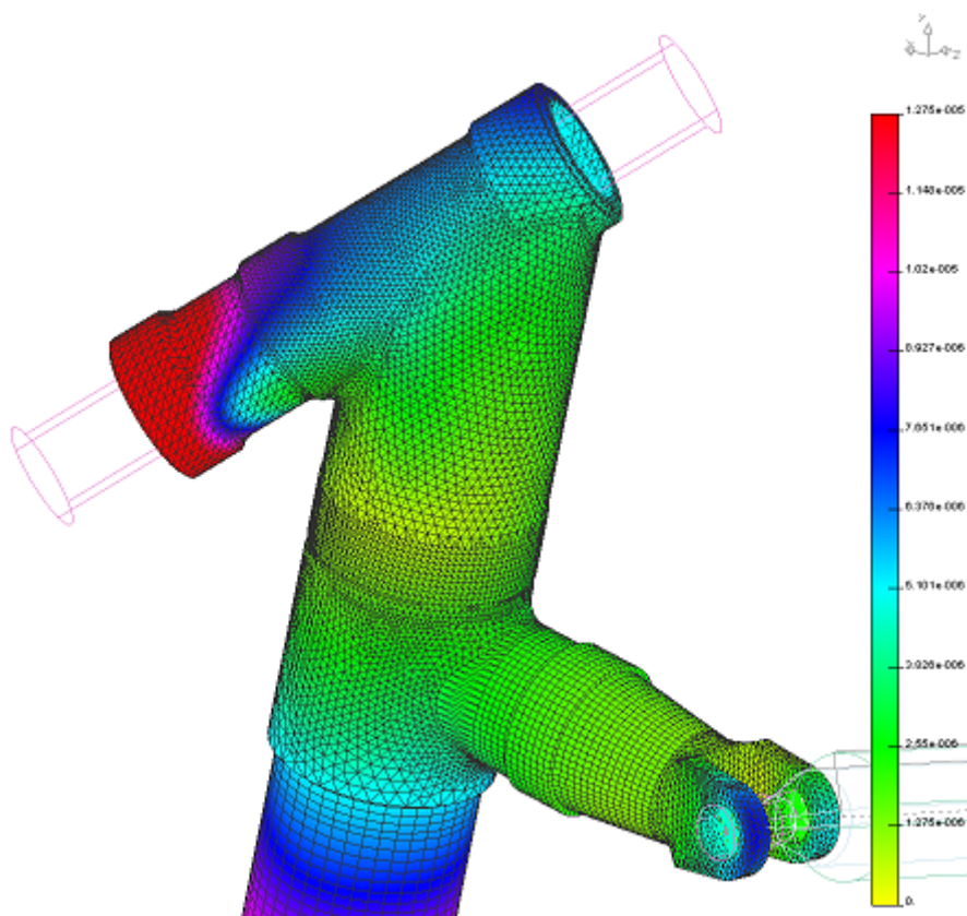
Рисунок 8. Деформации верхней части корпуса стойки
