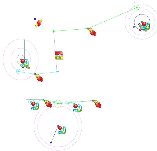
Рис. 3. Модель механизма автомата приемистости (АП)
