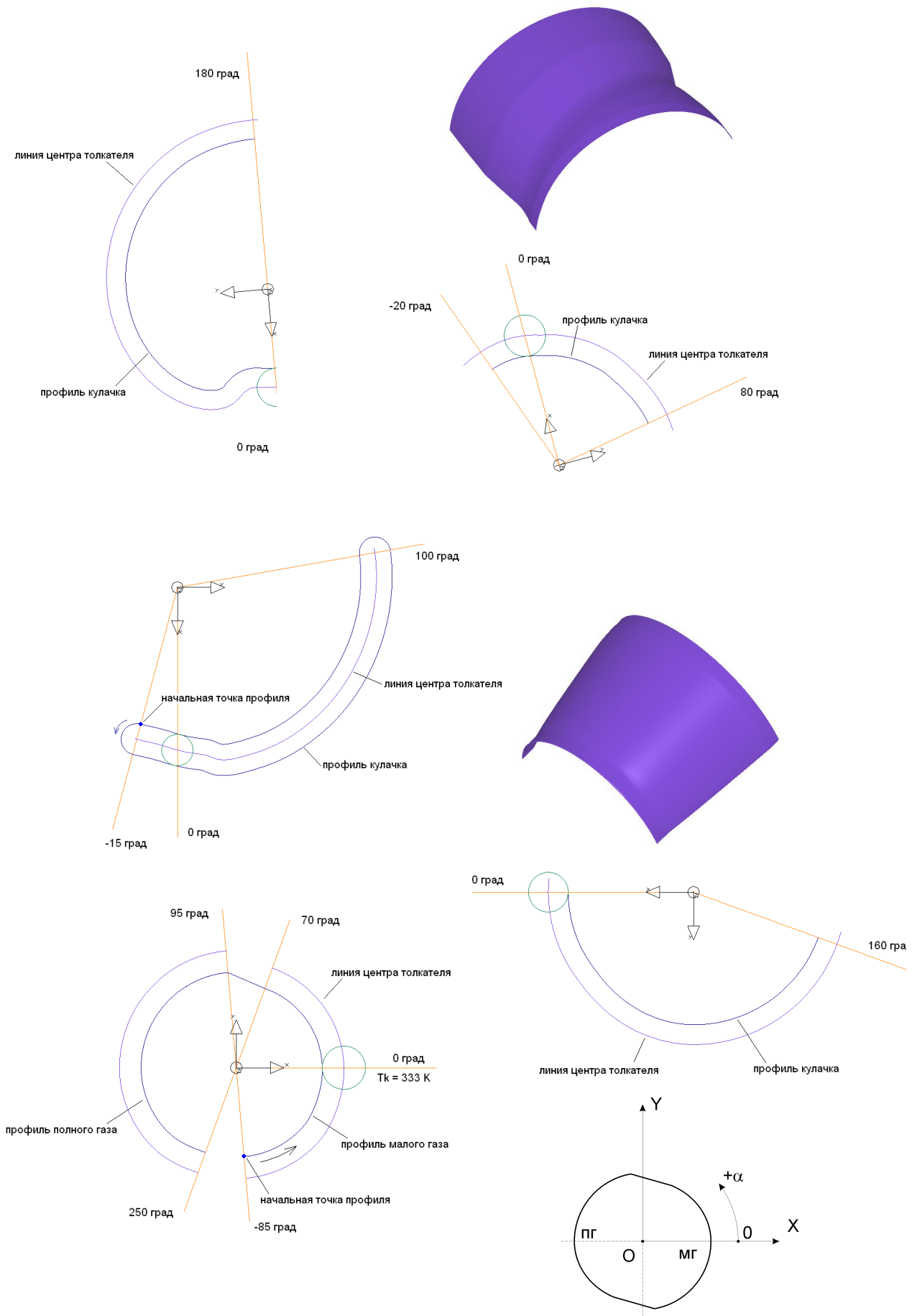
Рис. 5. Полученные профили кулачков
