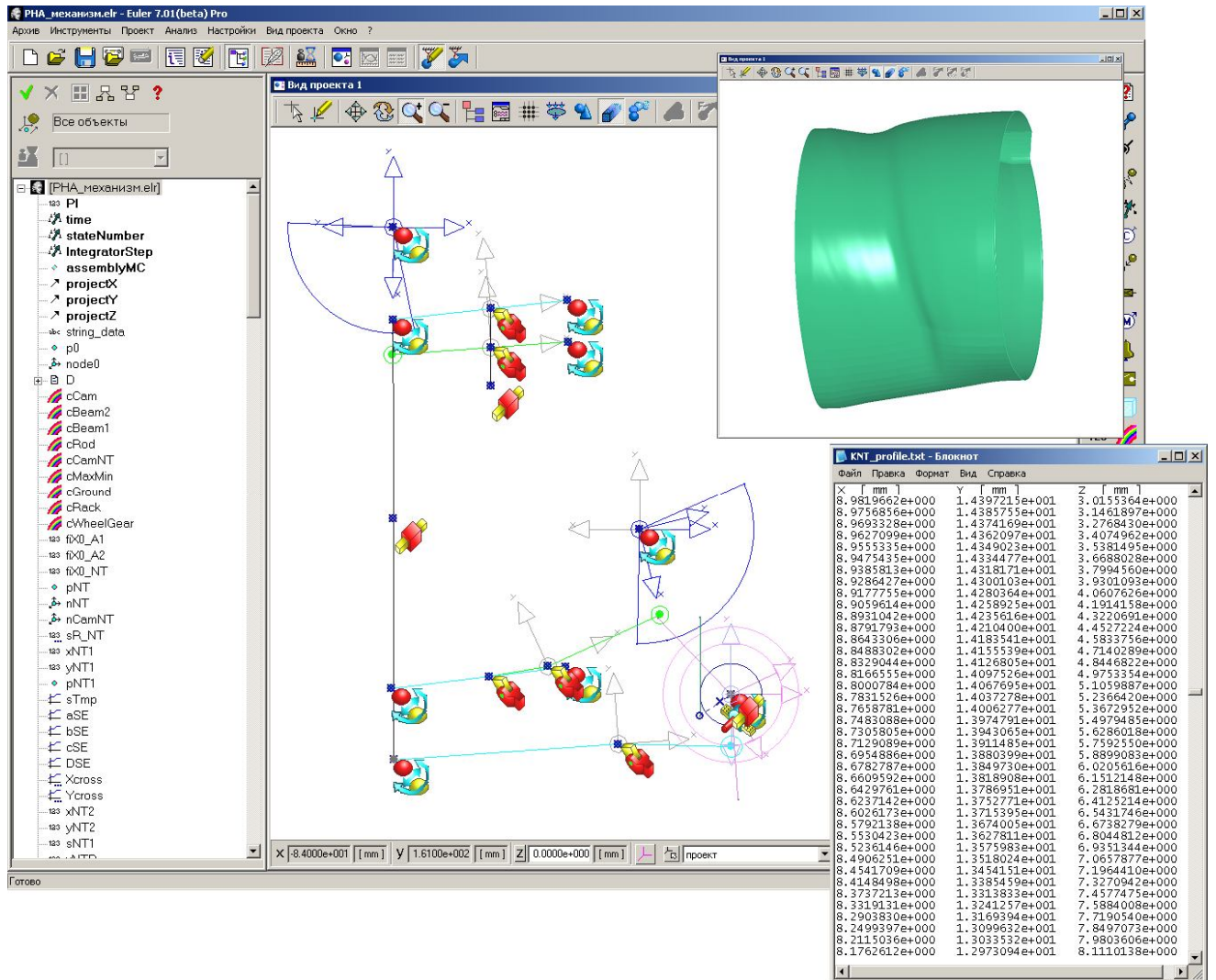
Рис. 6. Внешний вид экрана программного комплекса EULER
