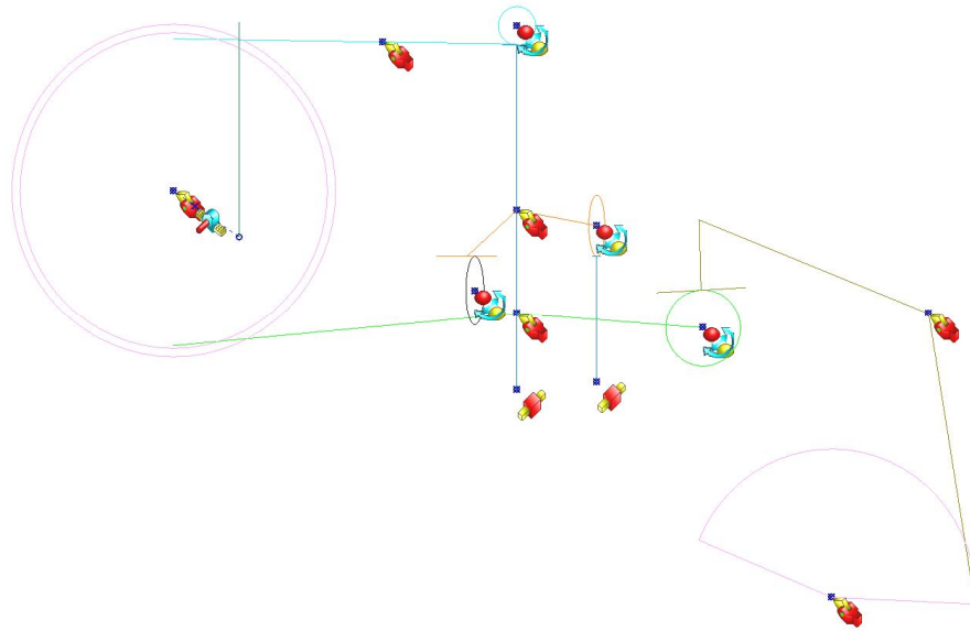
Рис. 2. Модель механизма регулятора оборотов (РО)
